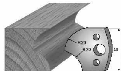
SP-Messer/Blade = Art.-Nr./Item no. 36120 HS-Messer/Blade = Art.-Nr./Item no. 36420 Abweiser/Deflector = Art.-Nr./Item no. 37120
