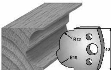
SP-Messer/Blade = Art.-Nr./Item no. 36115 HS-Messer/Blade = Art.-Nr./Item no. 36415 Abweiser/Deflector = Art.-Nr./Item no. 37115
