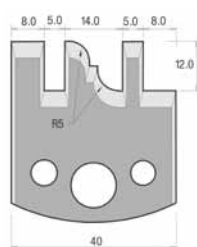
SP-Messer/Blade = Art.-Nr./Item no. 36137 HS-Messer/Blade = Art.-Nr./Item no. 36437 Abweiser/Deflector = Art.-Nr./Item no. 37137
