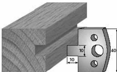
SP-Messer/Blade = Art.-Nr./Item no. 3691 HS-Messer/Blade = Art.-Nr./Item no. 36391 Abweiser/Deflector = Art.-Nr./Item no. 3791
