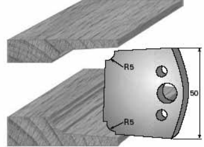
SP-Messer/Blade = Art.-Nr./Item no. 38579 HS-Messer/Blade = Art.-Nr./Item no. 36579 Abweiser/Deflector = Art.-Nr./Item no. 39579
