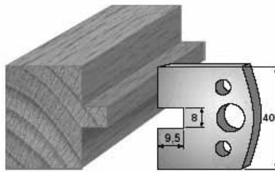
SP-Messer/Blade = Art.-Nr./Item no. 3695 HS-Messer/Blade = Art.-Nr./Item no. 36395 Abweiser/Deflector = Art.-Nr./Item no. 3795
