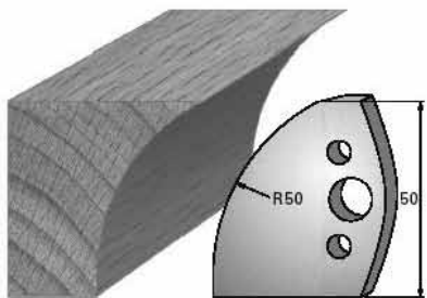
SP-Messer/Blade = Art.-Nr./Item no. 38567 HS-Messer/Blade = Art.-Nr./Item no. 36567 Abweiser/Deflector = Art.-Nr./Item no. 39567
