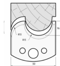
SP-Messer/Blade = Art.-Nr./Item no. 38539 HS-Messer/Blade = Art.-Nr./Item no. 36539 Abweiser/Deflector = Art.-Nr./Item no. 39539
