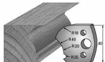
SP-Messer/Blade = Art.-Nr./Item no. 36123 HS-Messer/Blade = Art.-Nr./Item no. 36423 Abweiser/Deflector = Art.-Nr./Item no. 37123
